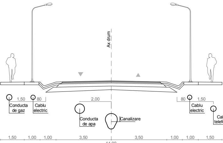
EXEMPLU PROFIL STRADAL CU AMPLASAREA ÎN LOCALITATE A REȚELOR EDILITARE SUBTERANE
